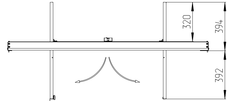
Исполнения ЦОД-СП-КОП-Нх-xxx.1500
