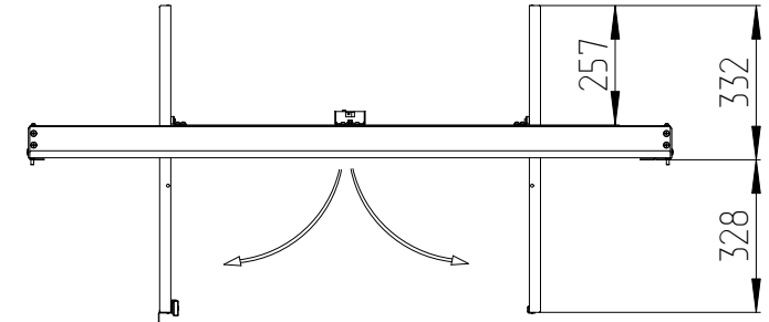
Исполнения ЦОД-СП-КОП-Нх-xxx.1250
